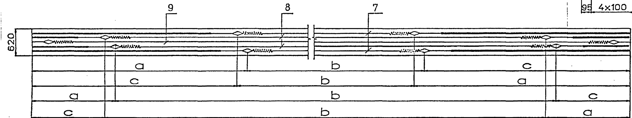
План второго арматурного ряда
