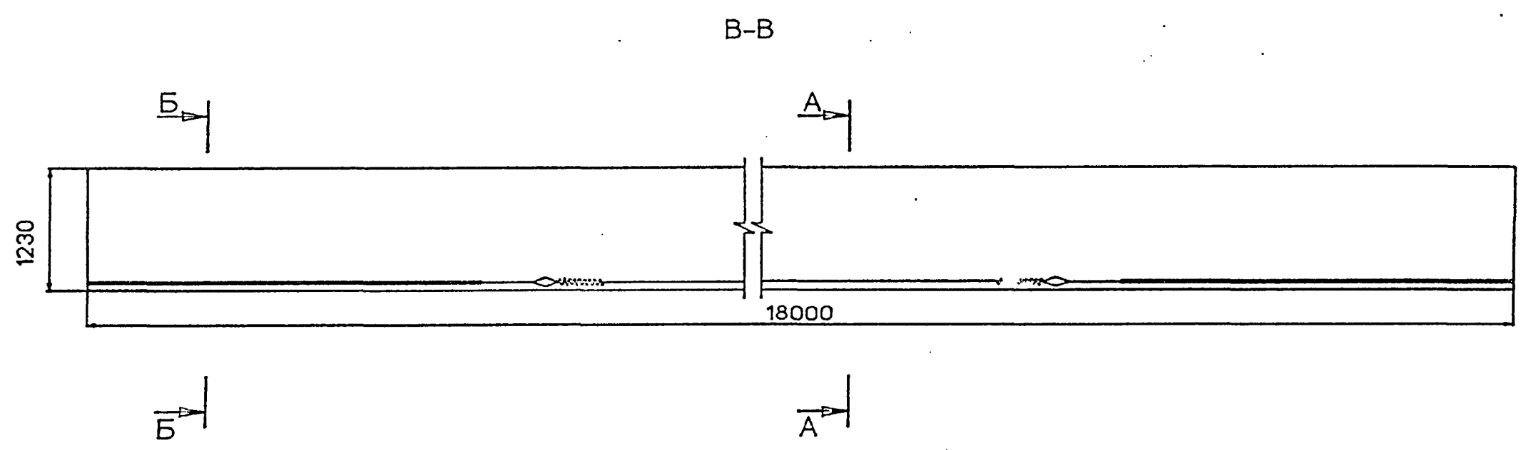
План первого арматурного ряда
