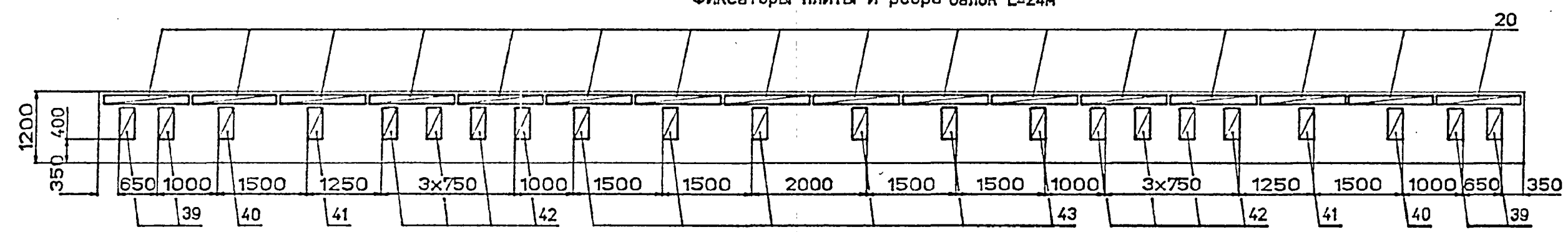
Фиксаторы плиты и ребра балок L=33м
