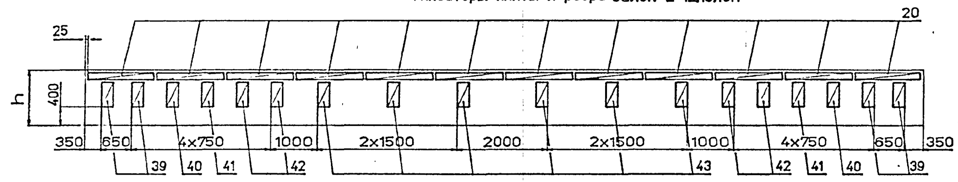
Фиксаторы плиты и ребра балок L=21м
