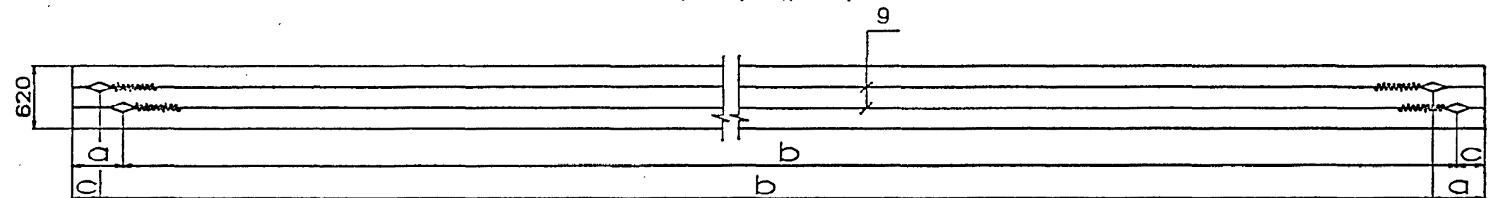
План второго арматурного ряда
