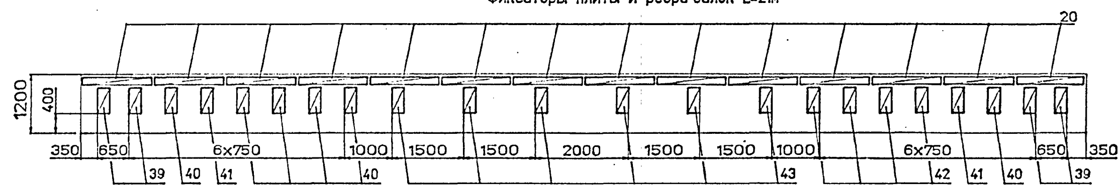
Фиксаторы плиты и ребра балок L=24м
