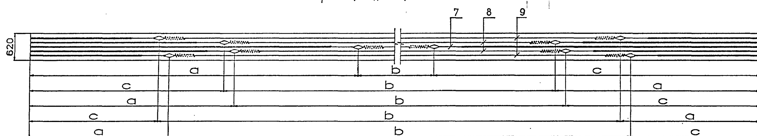
План первого арматурного ряда
