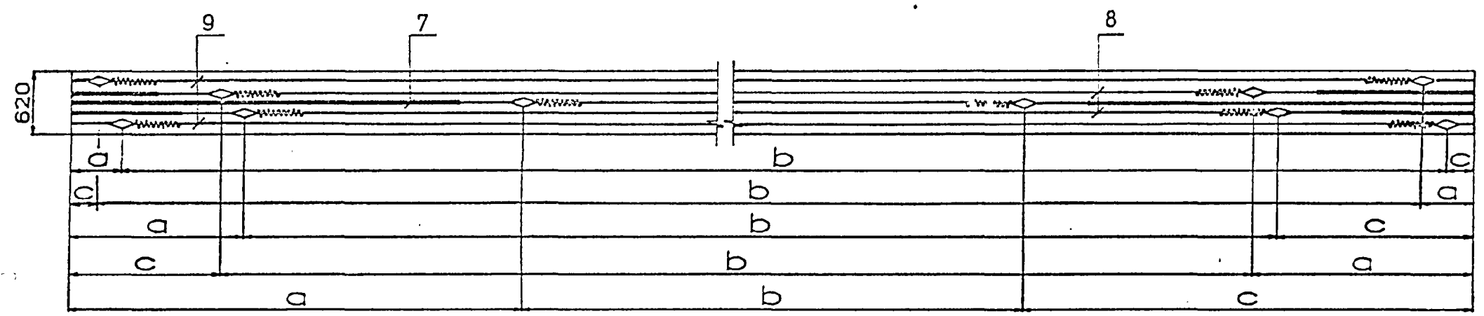
План первого арматурного ряда
