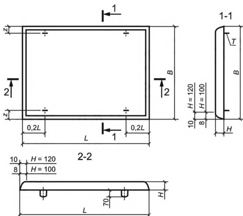
Рисунок А.1 — Плита типа 1П — для укладки в колее и междупутье на прямых участках пути
