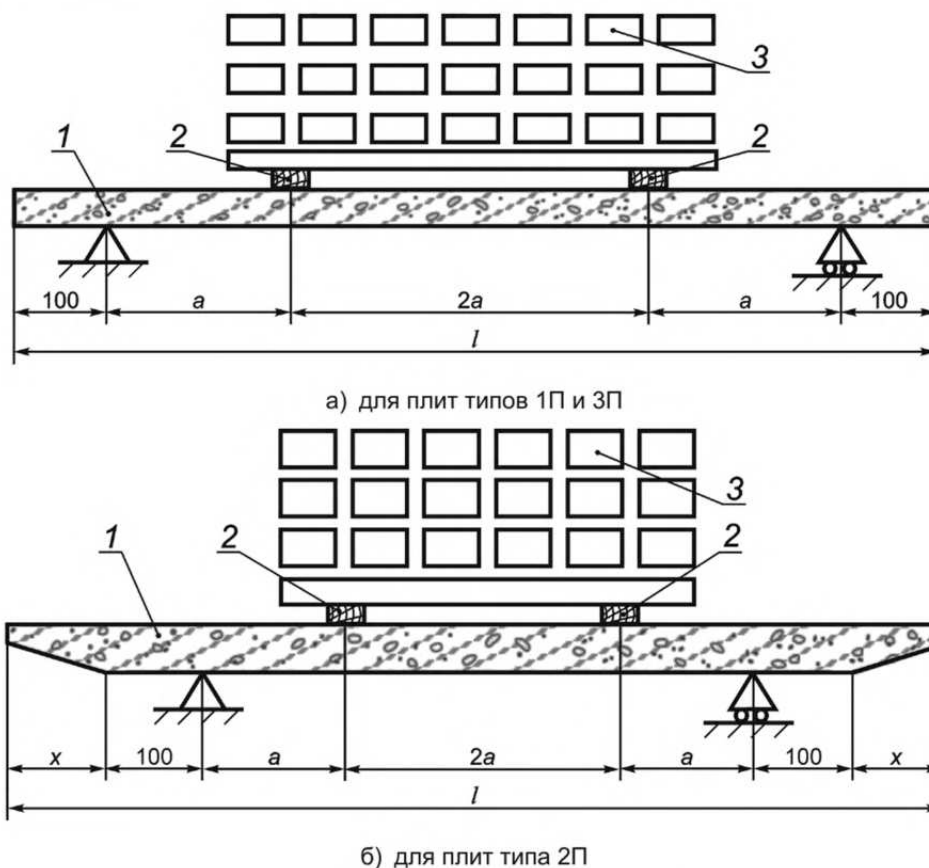
Рисунок 1 — Схемы испытаний плит
