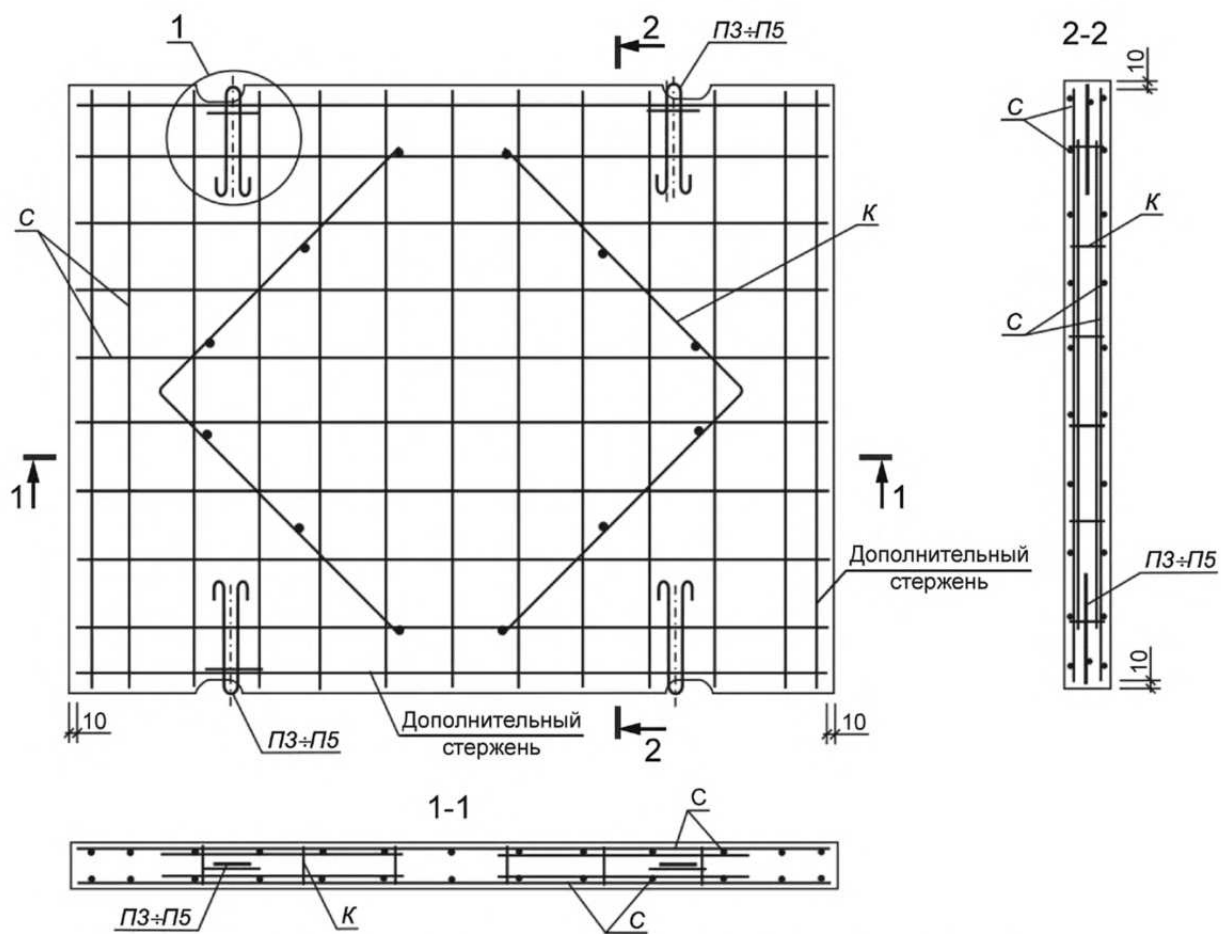
Рисунок В.1 — Схема армирования плит: П35.28, П30.18, П18.18, П18.15
