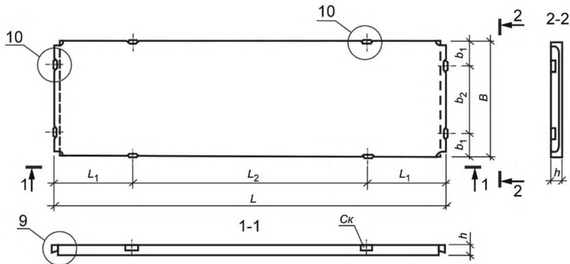
Рисунок А.16 — Плиты типов П и ПТ с пазами для беспетлевого монтажа
