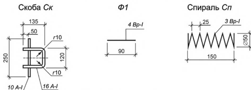
Рисунок Г.3 — Скоба Ск, спираль Сп, фиксатор Ф1
