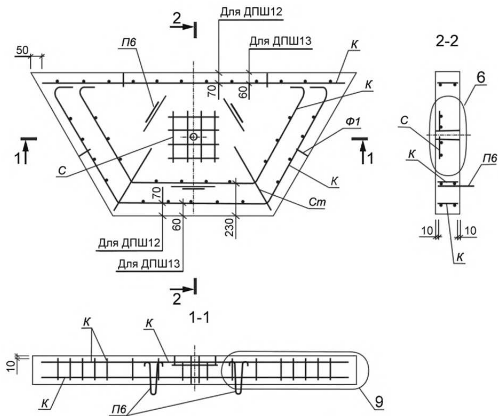
Рисунок В.5 — Схема армирования плит: ДПШ13, ДПШ12
