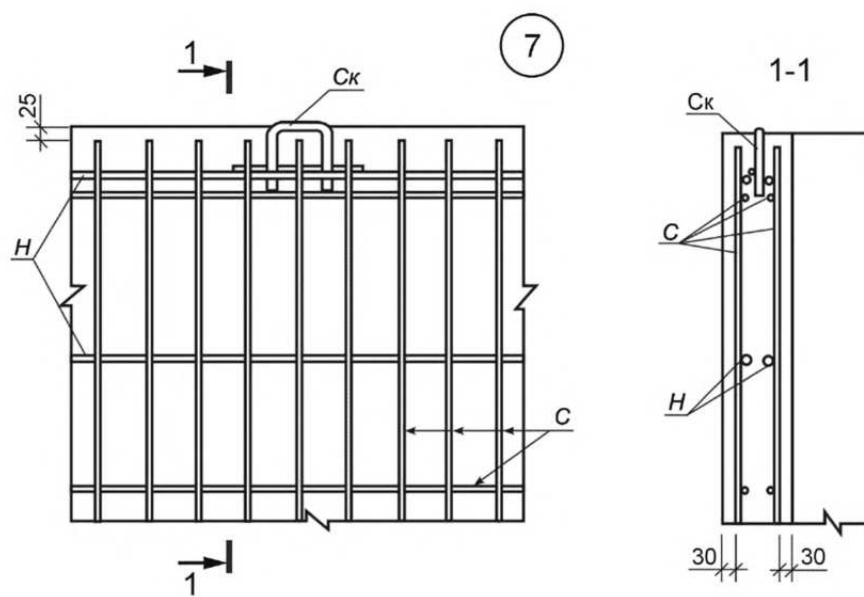
Рисунок Б.12 — Узел армирования 7
