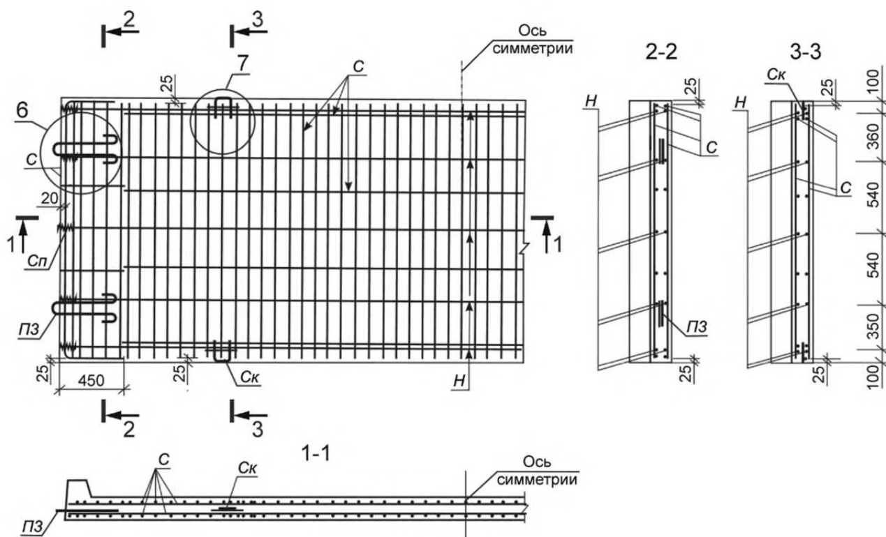
Рисунок Б.4 — Схема армирования плиты ПББ55.20
