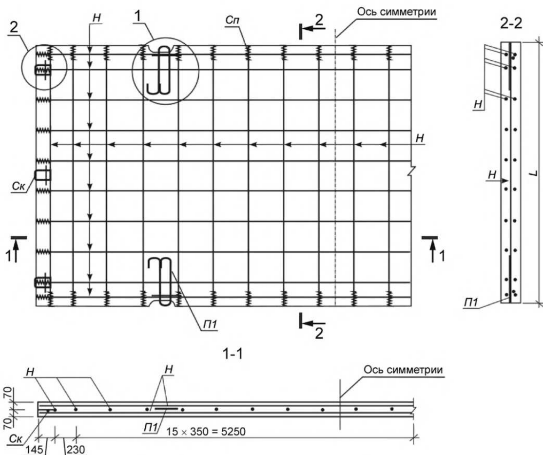
Рисунок Б.1 — Схемы армирования плит П60.38, П60.35, П60.30
