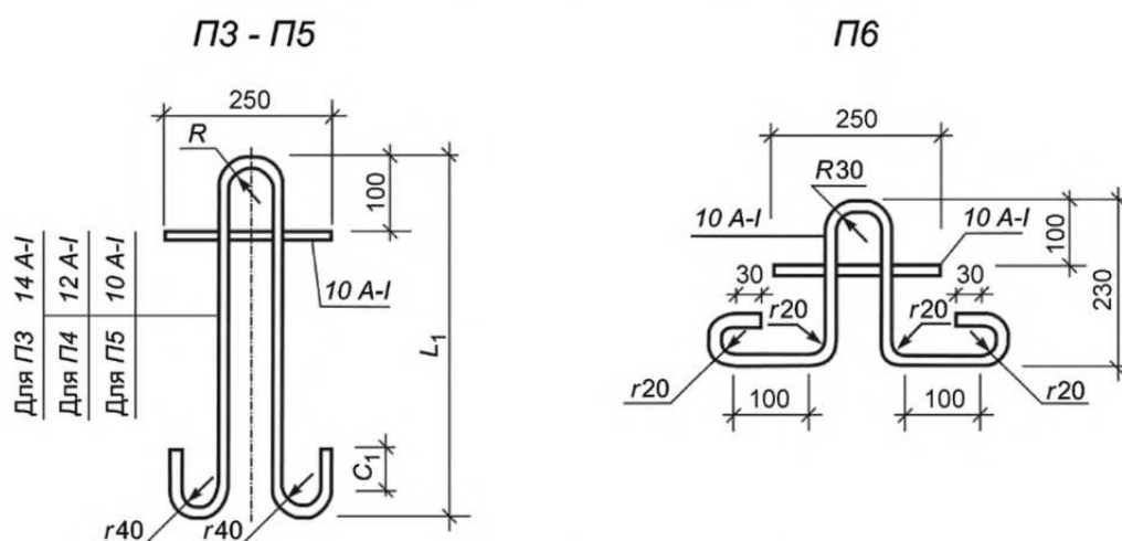
Рисунок Г.2 — Монтажные петли П3+П6
