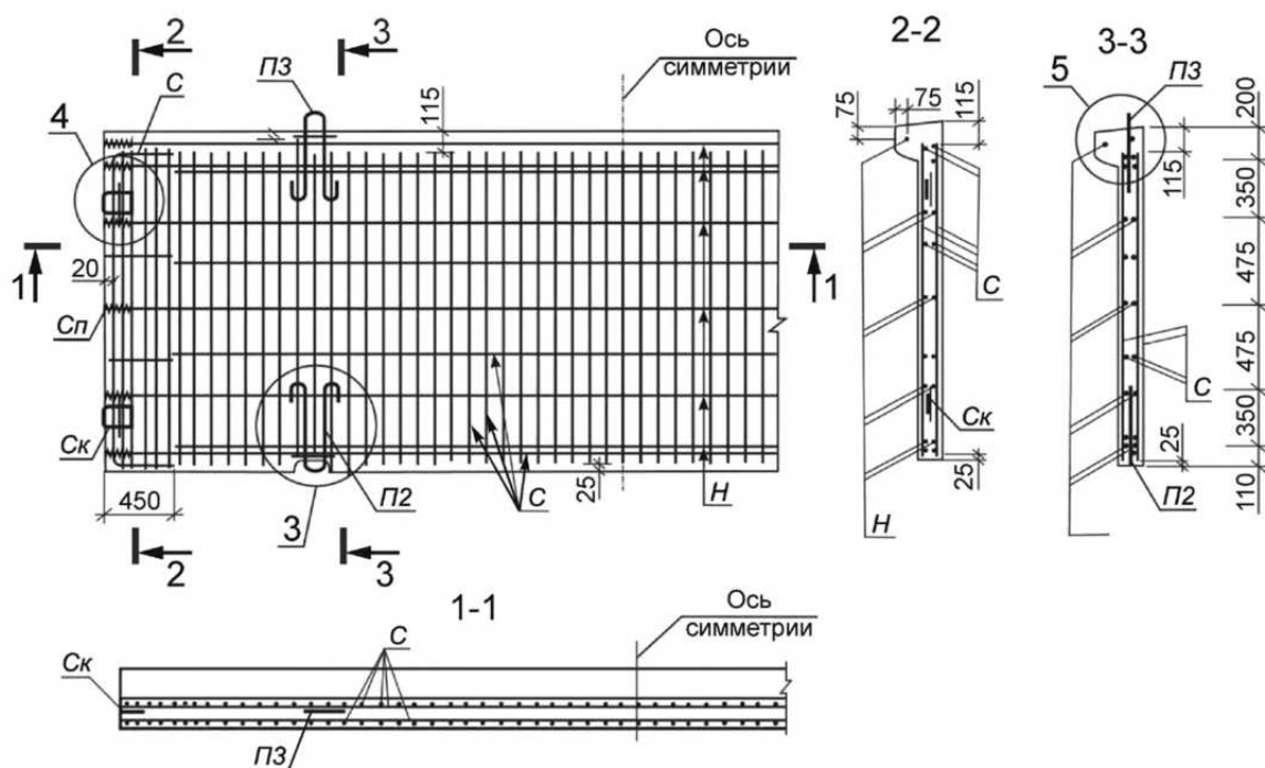
Рисунок Б.3 — Схема армирования плиты ПБ60.18
