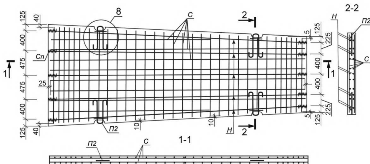
Рисунок Б.5 — Схема армирования плиты ПТ55
