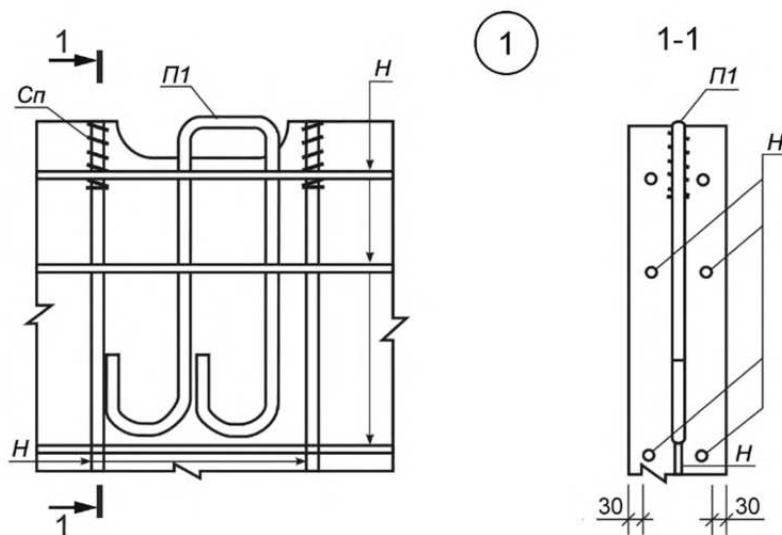
Рисунок Б.6 — Узел армирования 1
