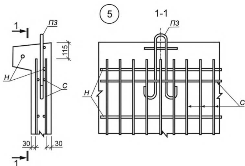
Рисунок Б.10 — Узел армирования 5
