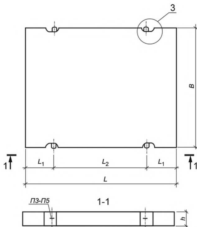
Рисунок А.3 — Плиты П35.28, П30.18, П18.18, П18.15
