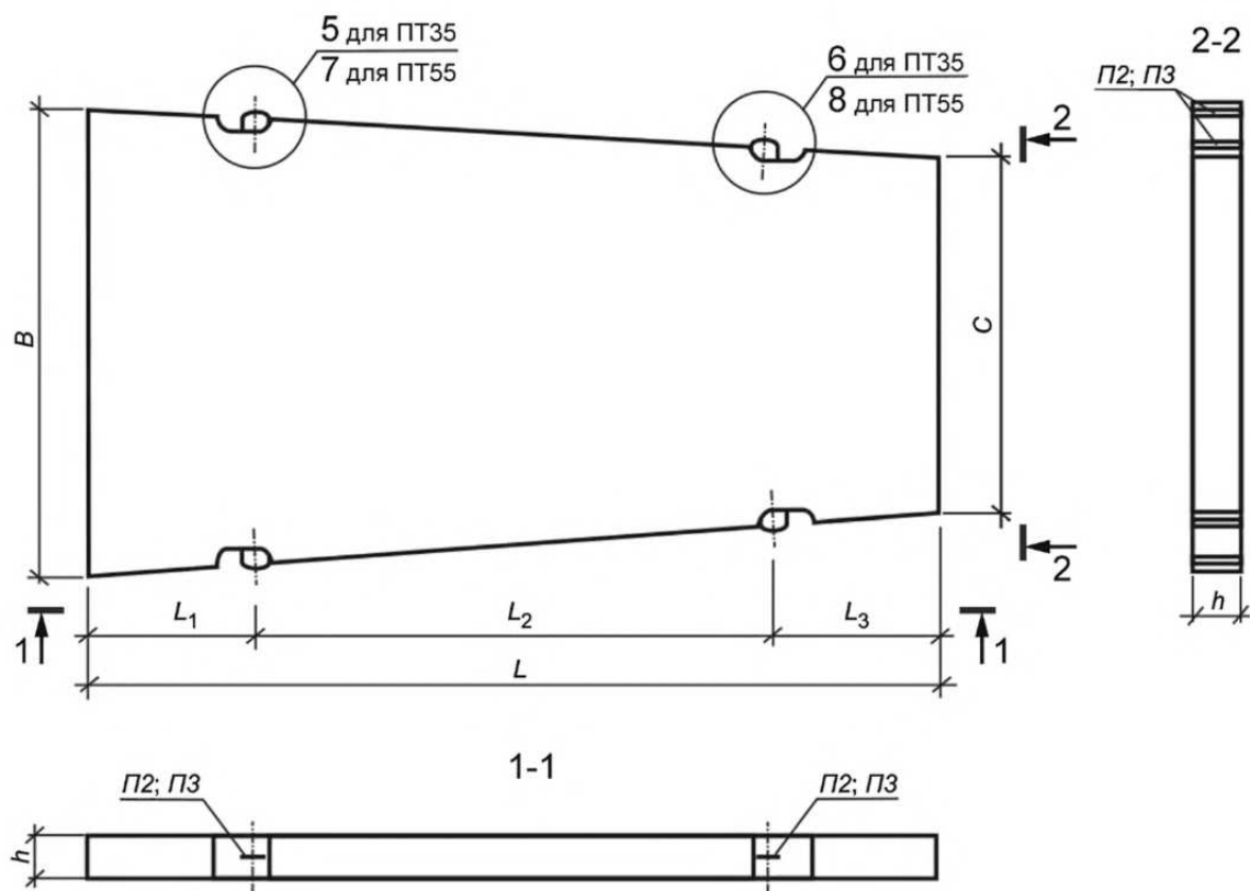
Рисунок А.6 — Плита ПТ
